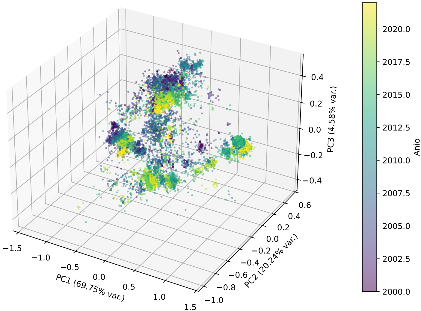
PCA 3D del espacio latente - por año
