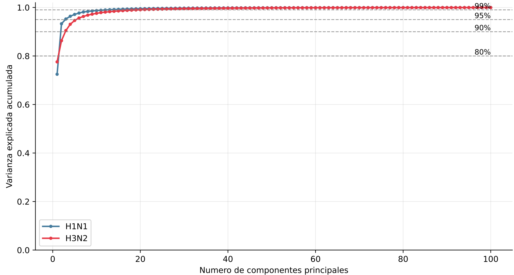
PCA por subtipo - varianza acumulada
