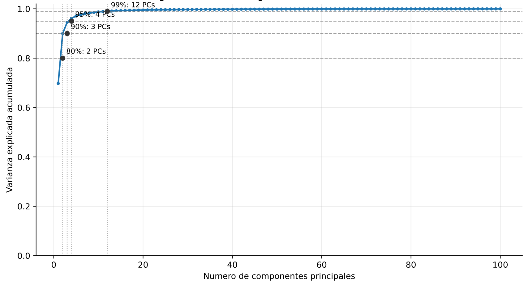
PCA global de embeddings latentes - varianza acumulada
