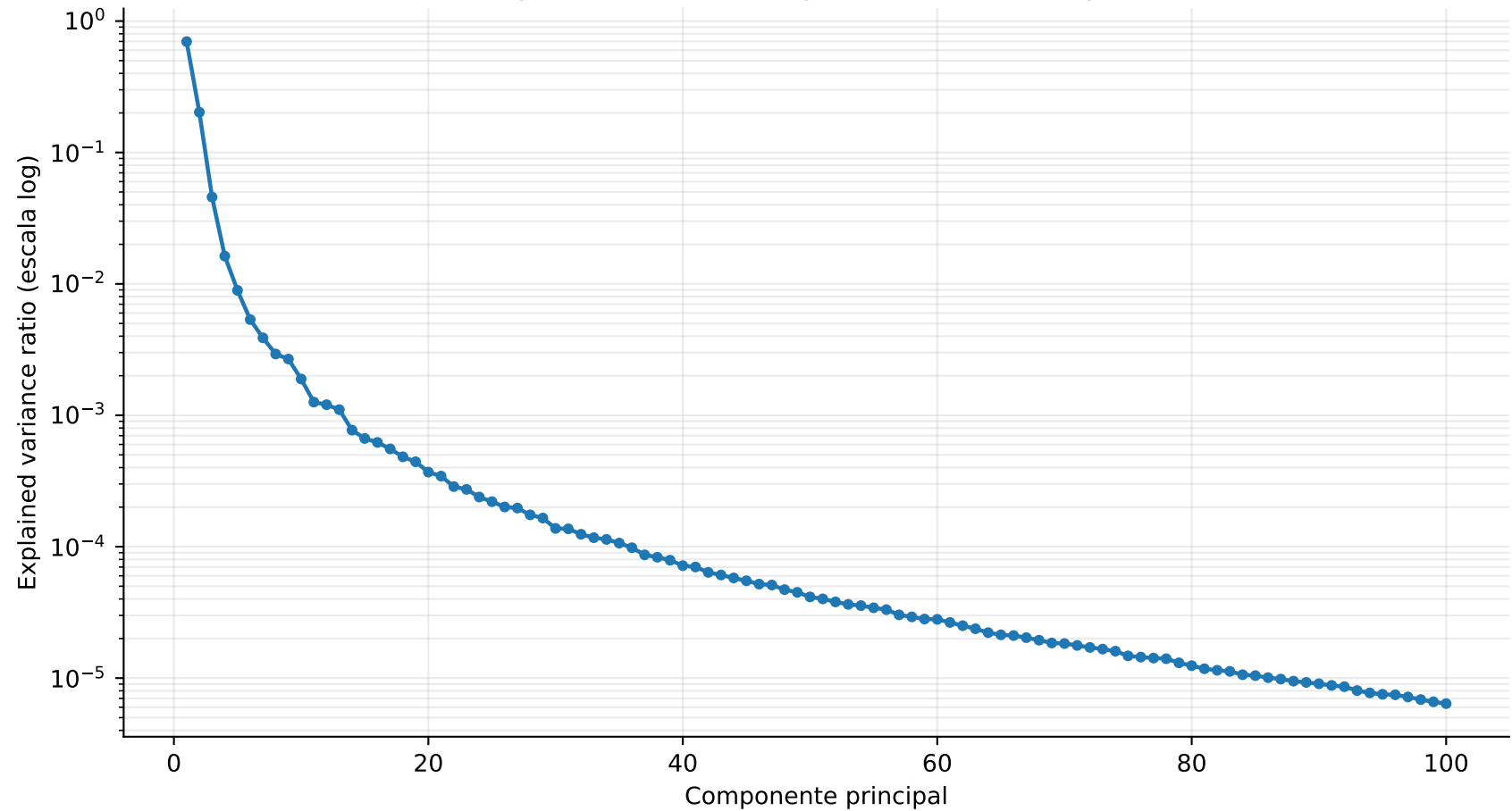
PCA global de embeddings latentes - cola espectral
