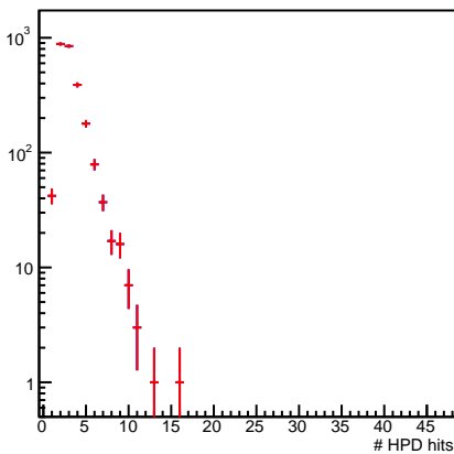
# HPD hits
