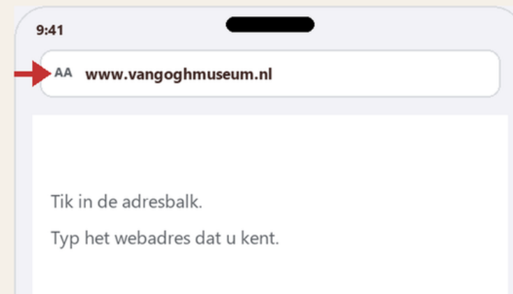
iPhone · Safari
