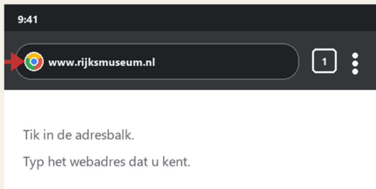
Android · Chrome
