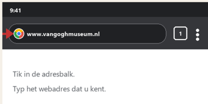
Android · Chrome
