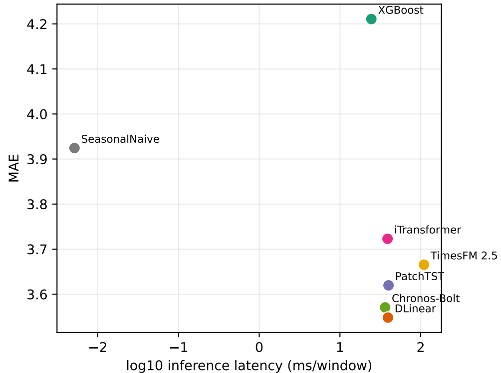
ETTH1
