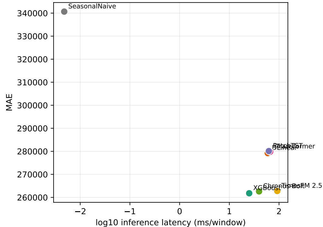
ECL
