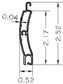
A1- E555 SLAT BLADE 6063-T6 Alloy
