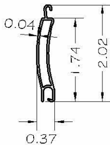
B1- E544 SLAT BLADE 6063-T6 Alloy
