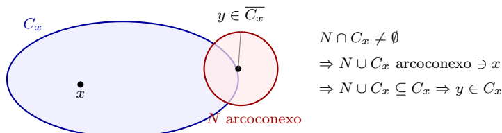
Figura 24. Por qué C_x es cerrada en un localmente arcoconexo (dibujo de la clase 12): un punto adherente y tiene un entorno arcoconexo N que pisa a C_x ; la unión es un arcoconexo que contiene a x , cabe en C_x , y arrastra a y con ella.
