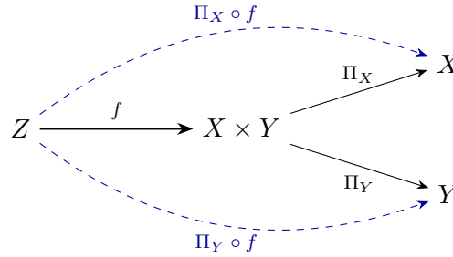
Figura 13. Una función hacia un producto es continua exactamente cuando sus dos coordenadas lo son. Es la propiedad universal del subespacio (§8) “para el otro lado”: allá la flecha auxiliar era la inclusión, que entra a X ; acá son las proyecciones, que salen del producto.
