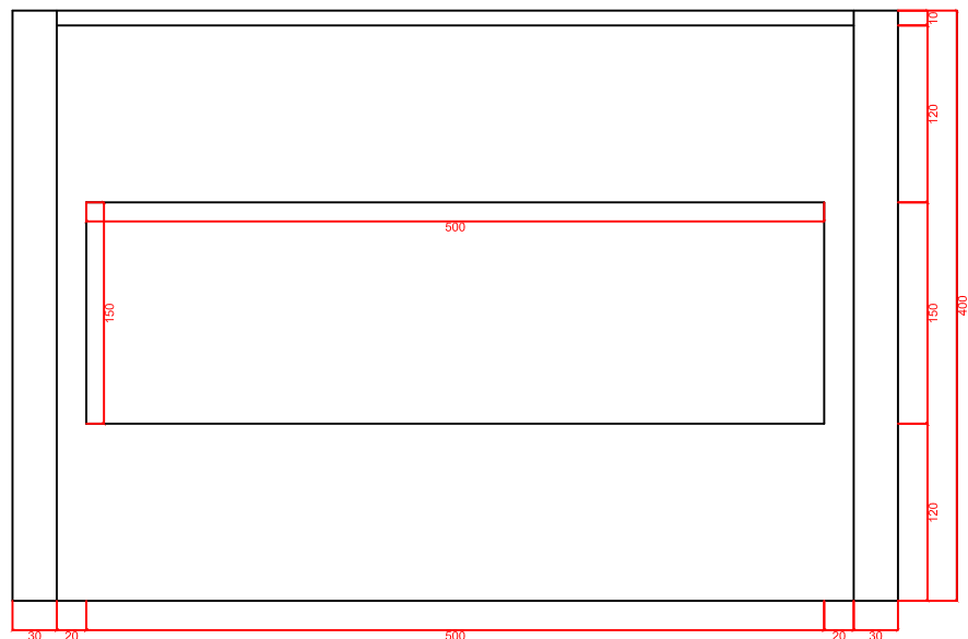
TAMPAK DEPAN
