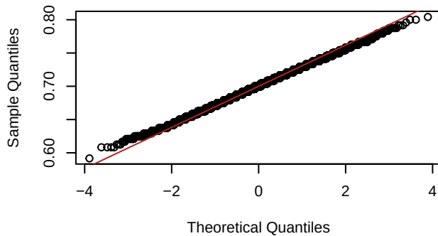
Q-Q Plot: n = 240
