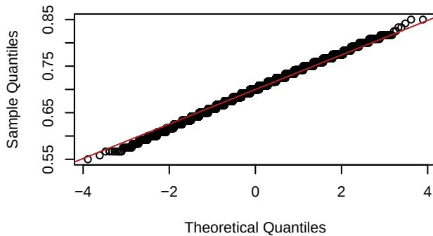
Q-Q Plot: n = 120
