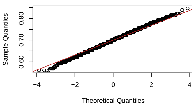
Q-Q Plot: n = 130
