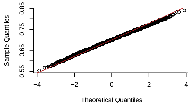
Q-Q Plot: n = 150
