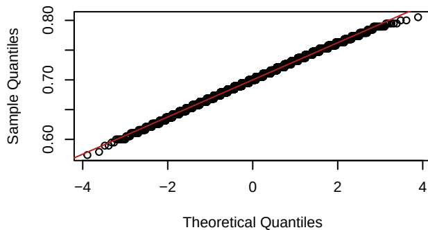
Q-Q Plot: n = 190
