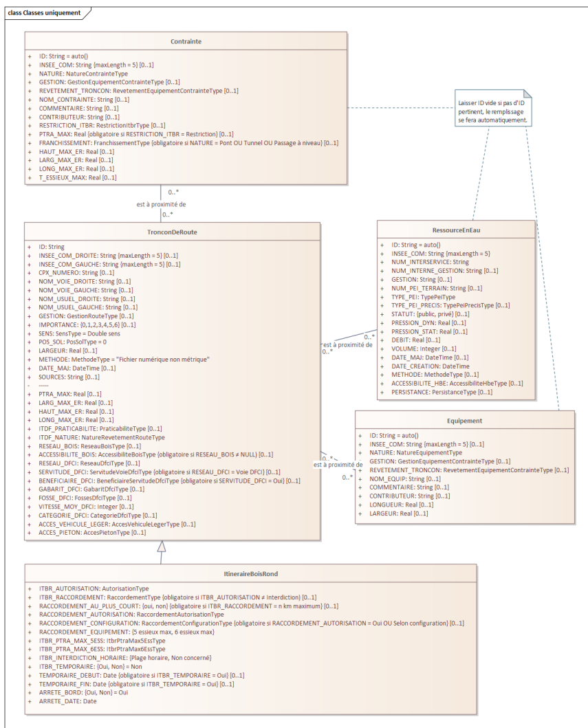
Figure 2 : Diagramme de classe (sans les énumérations)
