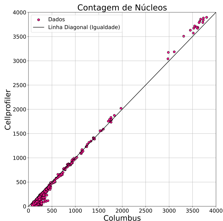
Figura 7: Gráfico de dispersão das contagens de núcleos do protocolo preliminar do CellProfiler e do software comercial Acapella/Columbus.
