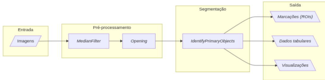
Figura 6: Fluxograma do protocolo preliminar de processamento de imagens em ensaios de viabilidade celular.
