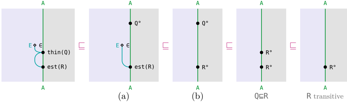
(a) \in \text{thin}(Q) \sqsubseteq Q^\circ \in — (14.1.1a)
