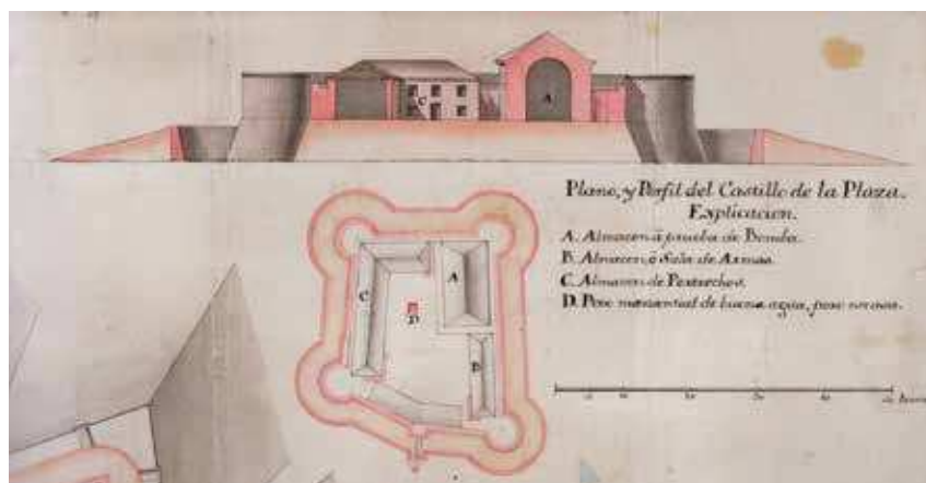
4.14 Alçado e planta do paiol barroco de Almeida, pormenor da planta de Almeida de António de Gaver, 15 de março de 1763 (Arquivo do Centro Geográfico del Ejército de Espanha)
