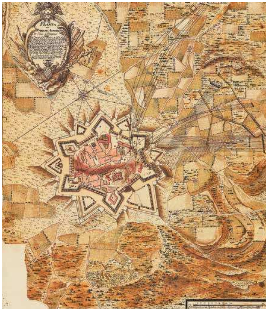
8.44 Planta de Almeida com os ataques, Luís Miguel Jacob, 1764 (Direção do Serviço de Infraestruturas do Exército)
