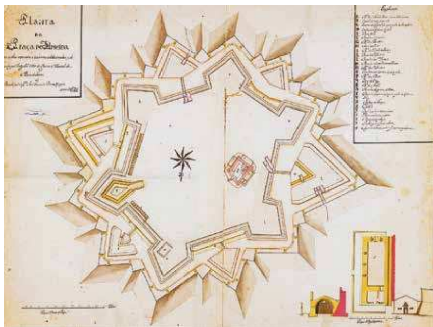
8.40 Planta de Almeida com as obras interiores e exteriores delineadas, Manuel de Azevedo Fortes e José Fernandes Pinto Alpoim, 1732 (c.) (Direção do Serviço de Infraestruturas do Exército)
