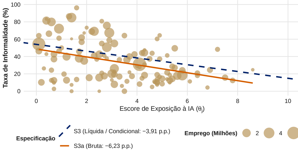
Figura 2: Mediação pela escolaridade da associação exposição–informalidade. Painel A: relação bruta (S3a, \hat{\delta}_1 = -6,23 p.p.; erro-padrão 0,99). Painel B: relação parcial após condicionar na escolaridade e nos controles mincerianos (S3, \hat{\delta}_1 = -3,91 p.p.; erro-padrão 0,96). A atenuação de 37,2% do coeficiente é consistente com a mediação parcial do Corolário 1.
