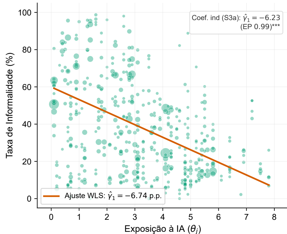
A. Relação Bruta (S3a: R^2 = 0.08 )
