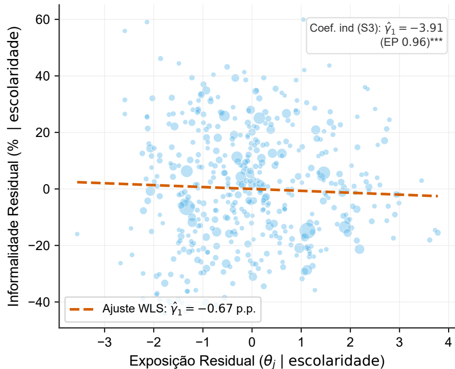
B. Regressão Parcial (S3: R^2 = 0.11 )
