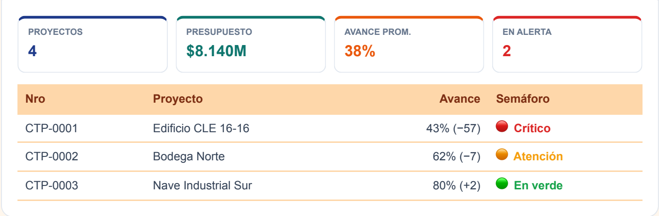
Figura 6. Portafolio — franja de totales + tabla con semáforo
