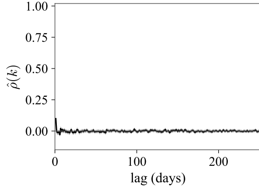
(D) Cross-sectional ACF of Daily Returns
