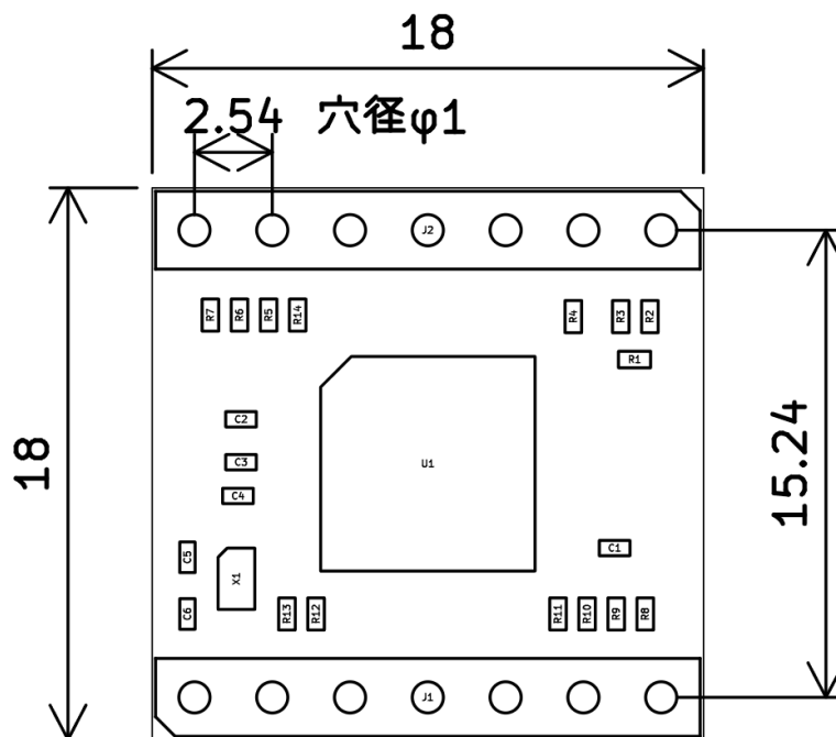
图 2：基板寸法图
