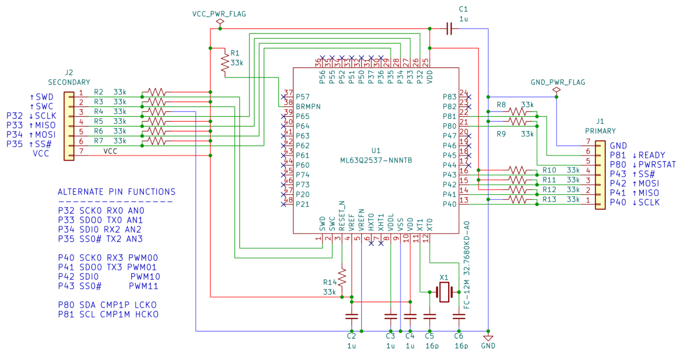
图 3：回路图
