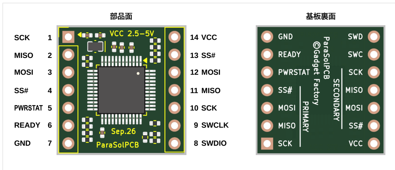
図 1: ピン配置図
