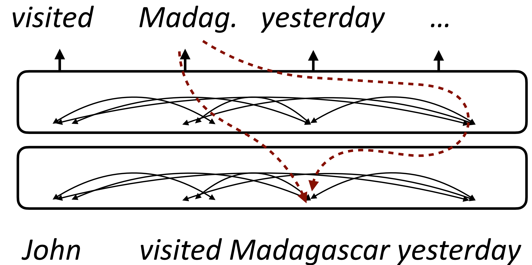
BERT
