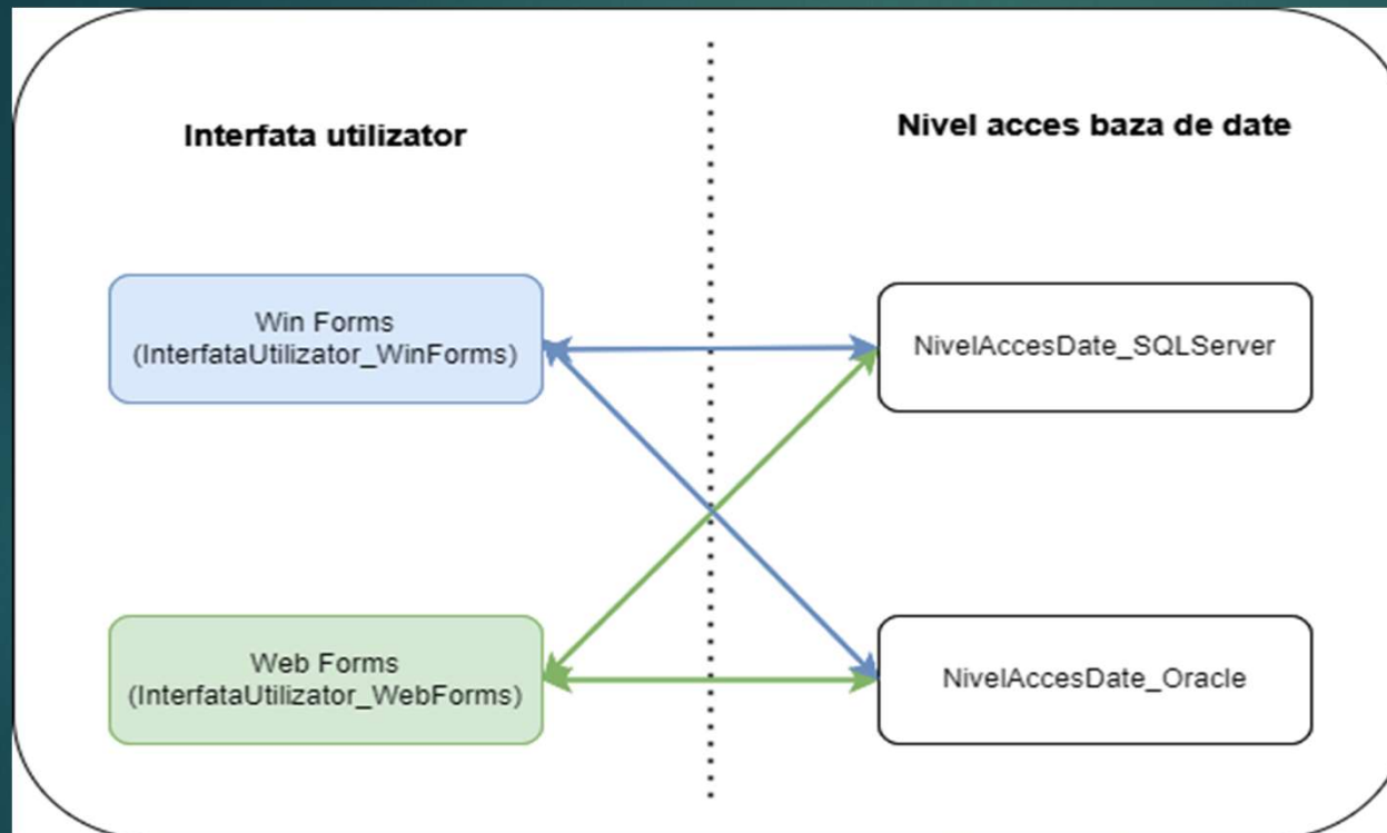
► Figura 2. Arhitectura aplicatiei demo
