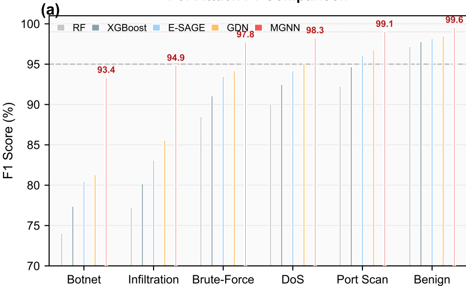
Per-Attack F1 Comparison
