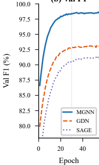
(b) Val F1
