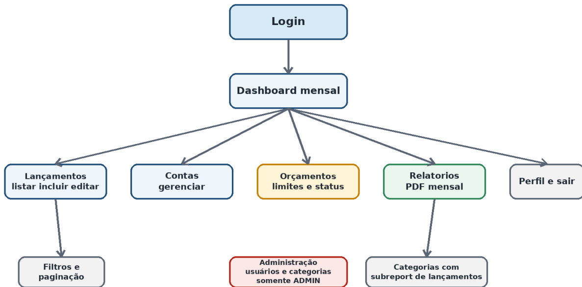
Figura 3 Navegação principal e separação da área administrativa
