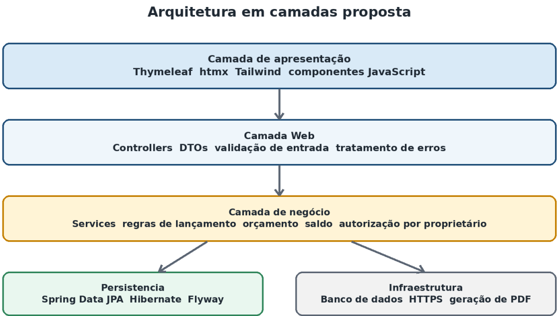
Figura 4 Arquitetura em camadas coerente com as etapas do trabalho
