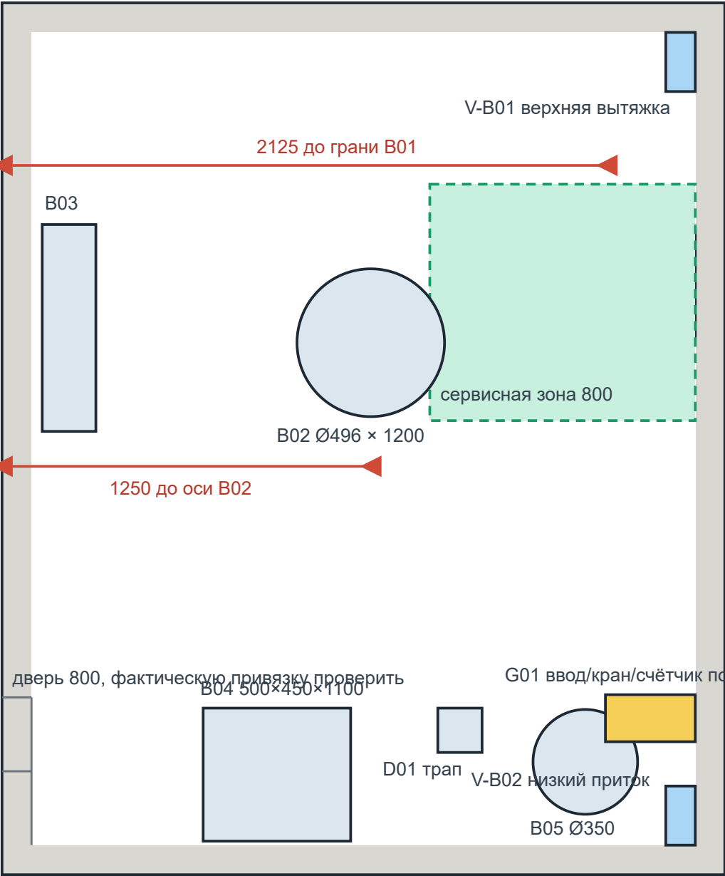
План, вид сверху
