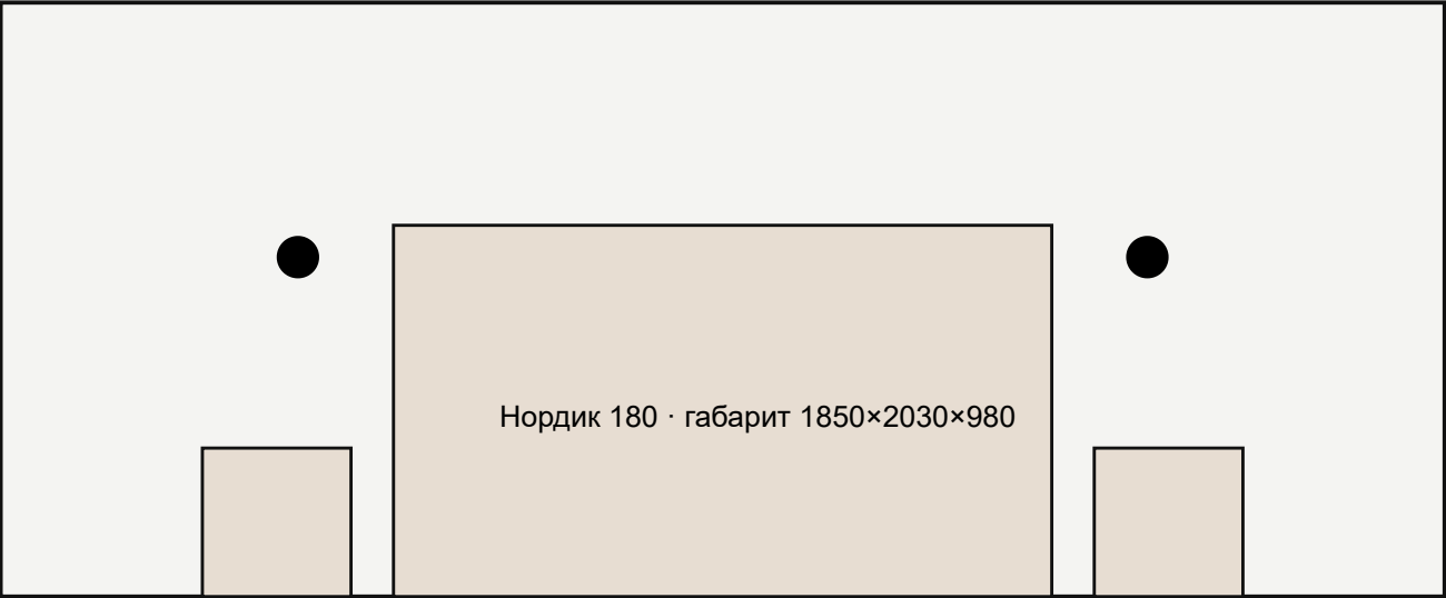
А. Стена изголовья, L=4430
