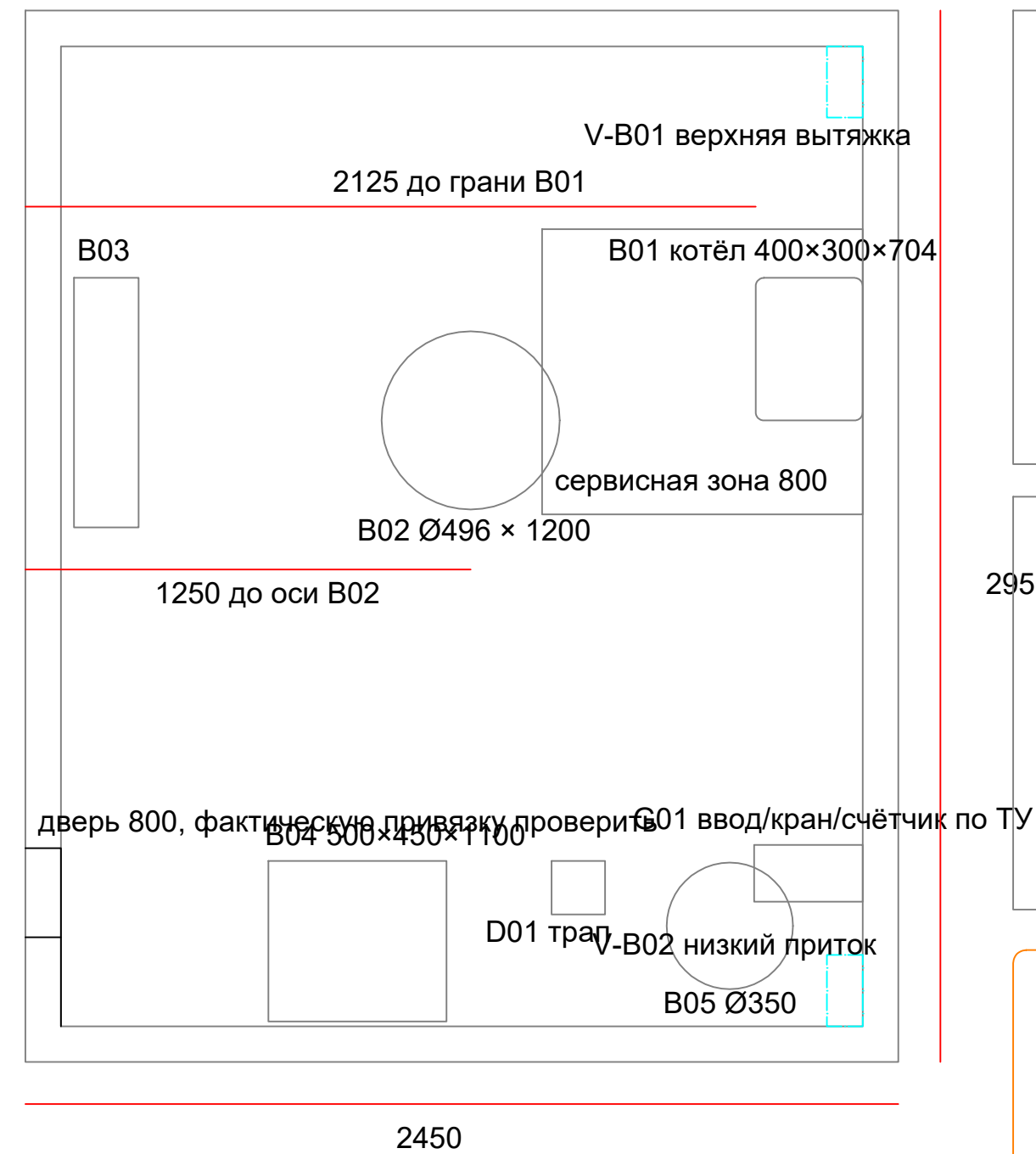
План, вид сверху
