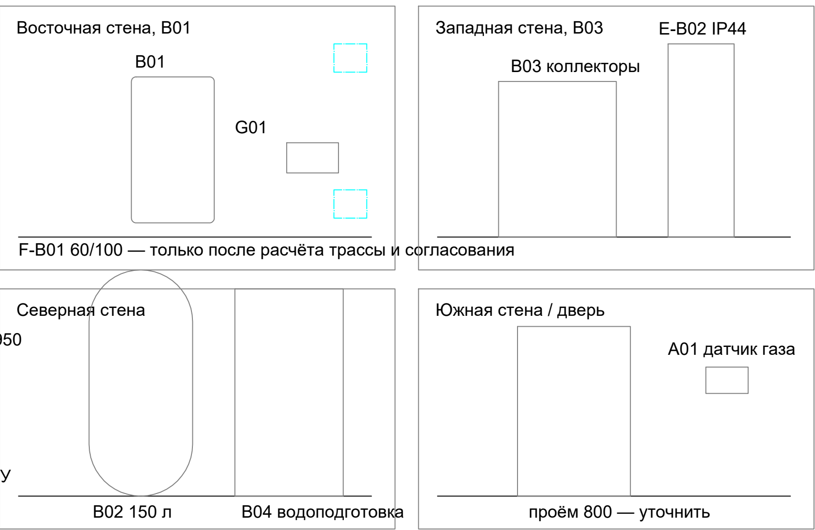
Развёртки стен — те же координаты C4D
