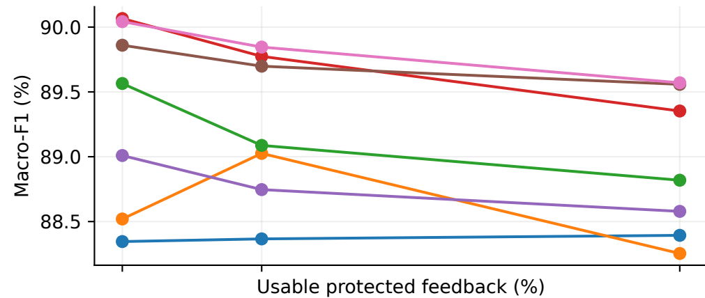
D3 OOF
