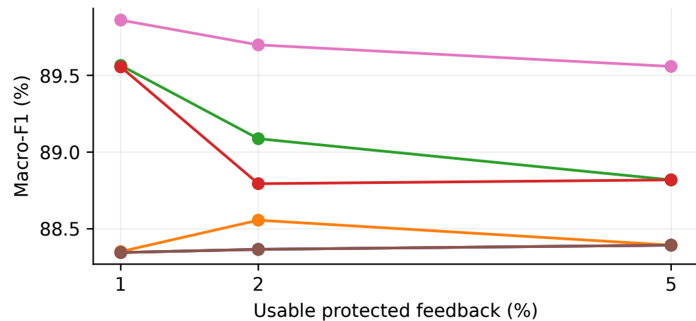
D3 OOF
