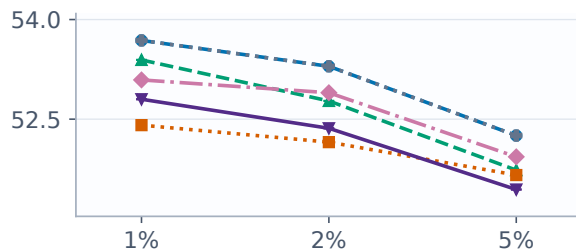
Macro-F1 (%)
