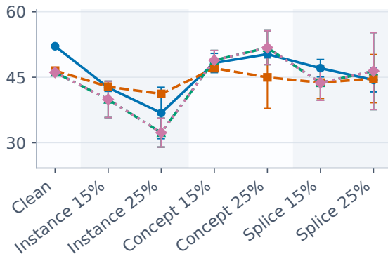
Macro-F1 (%)
