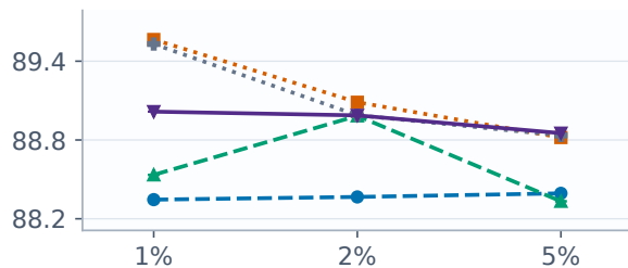
Macro-F1 (%)
