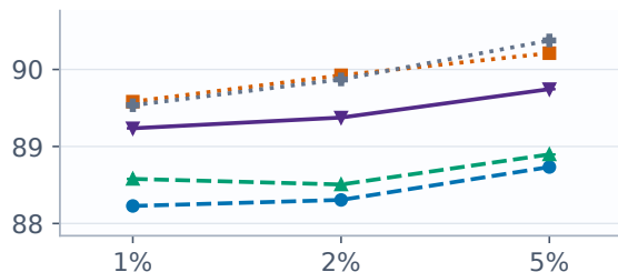
Macro-F1 (%)
