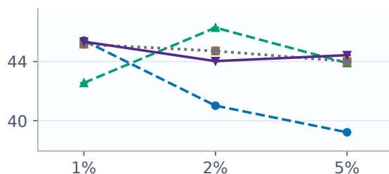
Macro-F1 (%)
