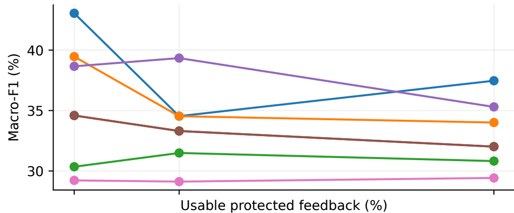
D3 OOF
