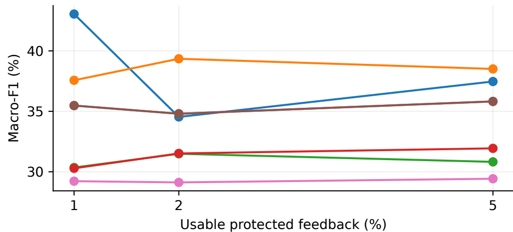
D3 OOF
