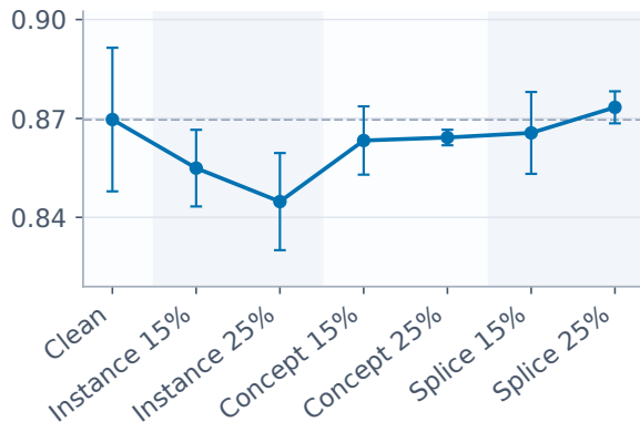
ROC-AUC
