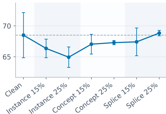
Macro-F1 (%)
