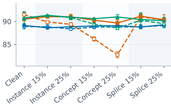
ROC-AUC
