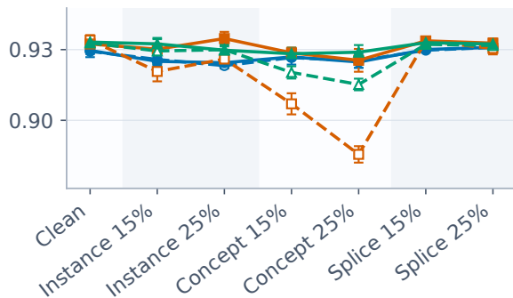
ROC-AUC
