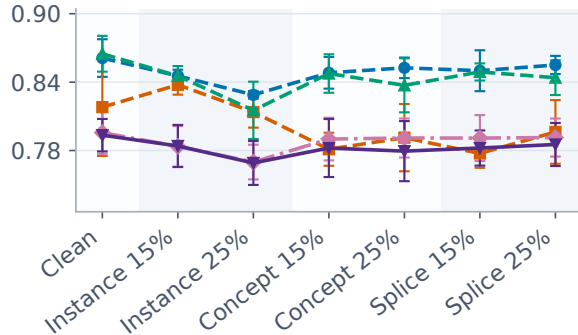
ROC-AUC
