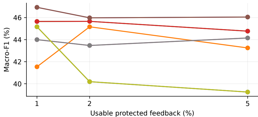
D3 OOF
