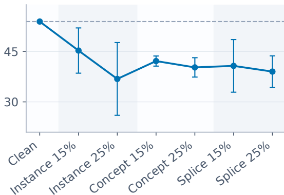
Macro-F1 (%)
