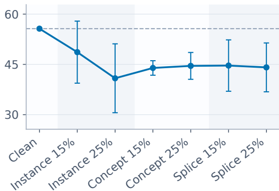
Macro precision (%)
