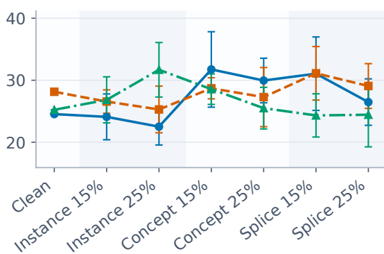
Macro-F1 (%)
