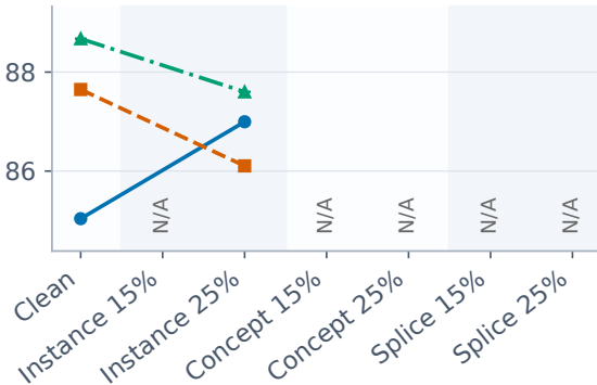
Macro-F1 (%)
