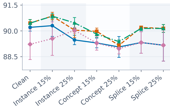
Macro-F1 (%)
