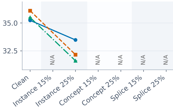
Macro-F1 (%)
