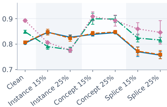
ROC-AUC
