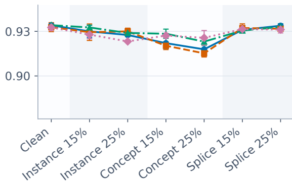
ROC-AUC
