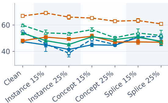
ROC-AUC
