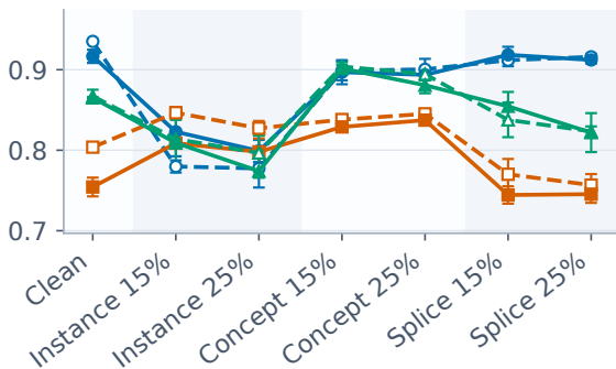
ROC-AUC
