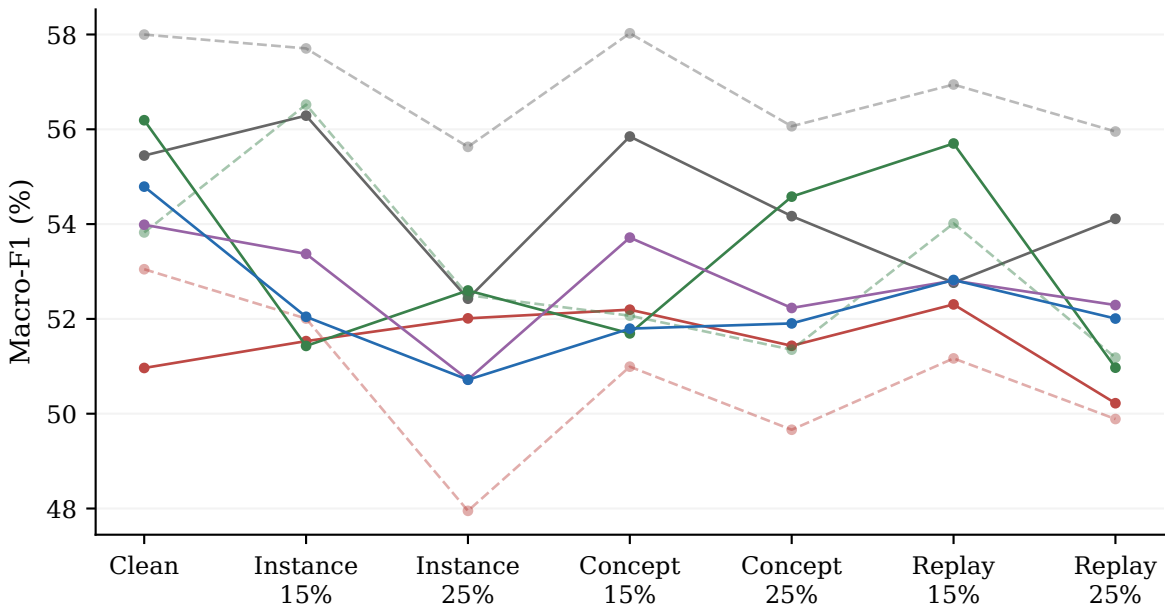
RBF, ADWIN: Macro-F1
