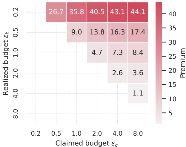
OUE premium, n=100k , d=32
