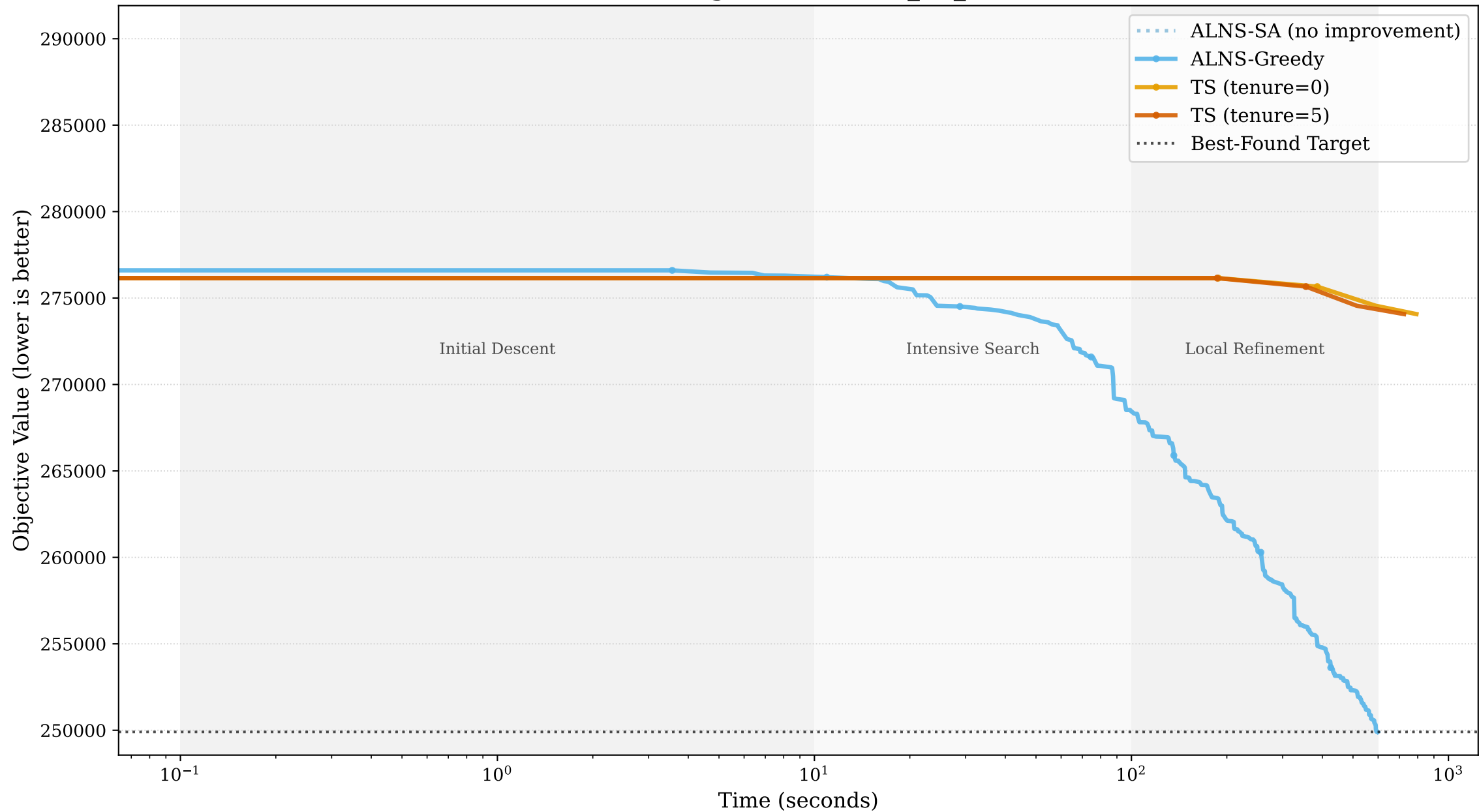
Convergence Plot: C1_10_2
