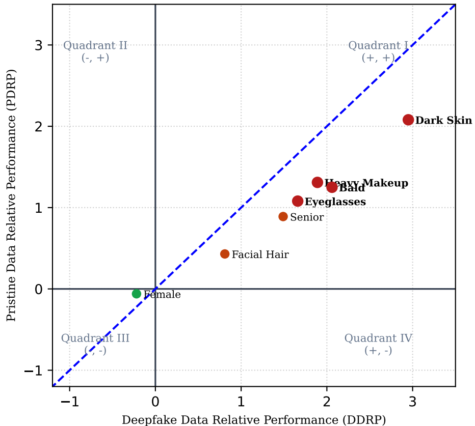
(b) Celeb-DF: Xception (PDRP vs. DDRP)
